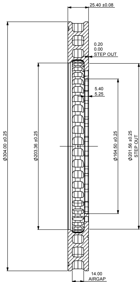
SECTION A-A
